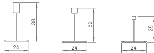
S 3 cliq / S 3a cliq Tragprofil Verbindungsprofil Verbindungsprofil
