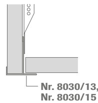
Deckenversprung oder Abschottung
