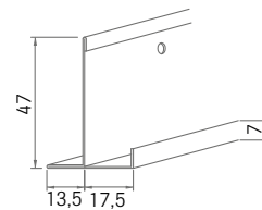
Nr. 8030/15 15er Platte 0,6 mm dick
