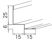
Nr. 50/14 0,5 mm dick
