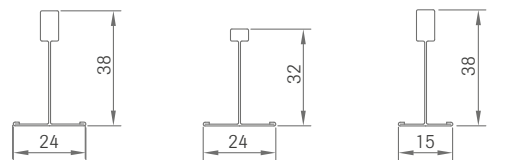
S 3 / S 3a Tragprofil Verbindungsprofil S 15 cliq / S 15a cliq Trag- und Verbindungsprofil
