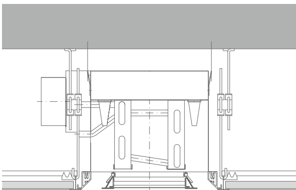
Klimatelement in OWA-Bandrastrerdecke integriert
