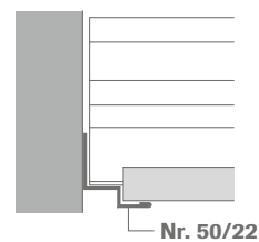
freigesp. Decken, z. B. Flurdecken mit Contura-Platten nach System S 6b
