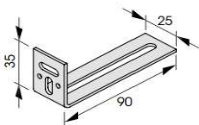
Wandanker WA
