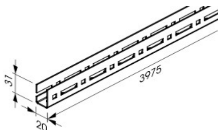
U-Profil GRID 20/30/20 gelocht Länge 3975 mm
