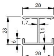
Tragprofil H-28 Länge 4000 mm
