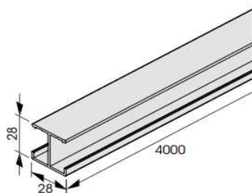
Tragprofil H-28 Länge 4000 mm
